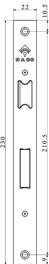
Front view Scale: 1:1
